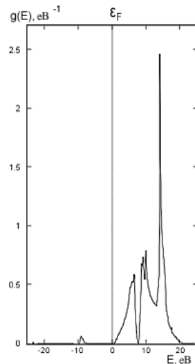
Рис. 7 – Вклад орбіталей атома \text{Mg} в щільність станів \text{MgO} у моделі \text{GGA} - \text{PBE} з урахуванням поправки Хабарда U = 7.86 \text{ eV} .
