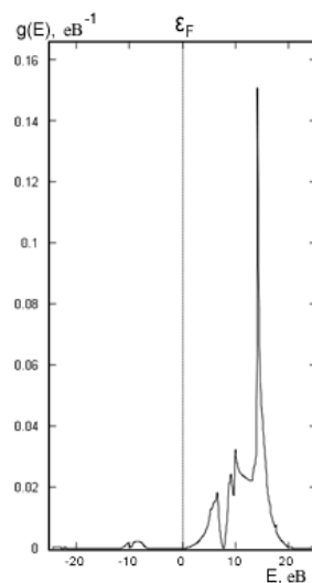
Рис. 13 – Вклад d-орбіталей атома О в щільність станів MgO в моделі GGA – PBE з урахуванням поправки Хабарда U = 7.86 eB.
