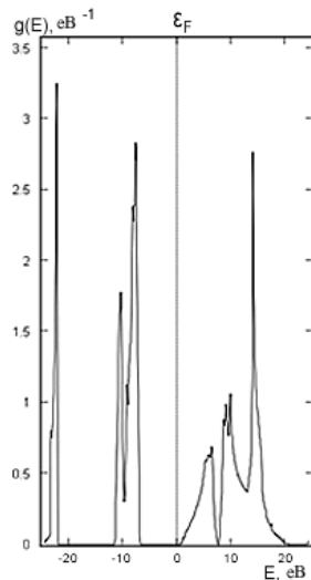
Рис. 6 – Щільність станів \text{MgO} в моделі \text{GGA} - \text{PBE} з урахуванням поправки Хабарда U = 7.86 \text{ eV} .
