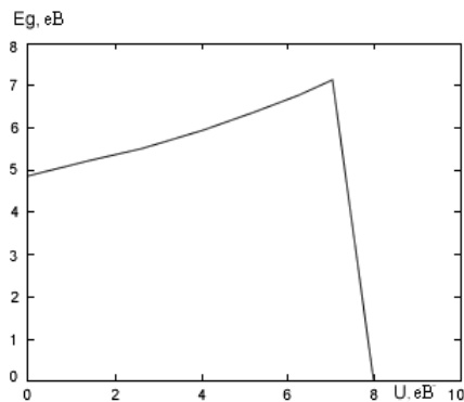
Рис. 2 – Залежність ширини E_g забороненої зони MgO в моделі GGA – PBE від величини параметра Хаббарда U в інтервалі 0 – 10 eV.
