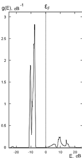
Рис. 12 – Вклад р-орбіталей атома О в щільність станів MgO в моделі GGA – PBE з урахуванням поправки Хабарда U = 7.86 eB.
