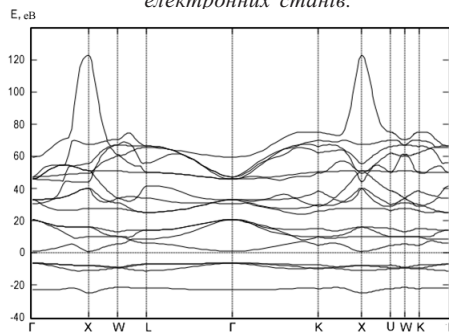
Рис. 5 – Зонна структура MgO в моделі GGA – PBE з поправкою Хабарда U = 7.86 eV.
