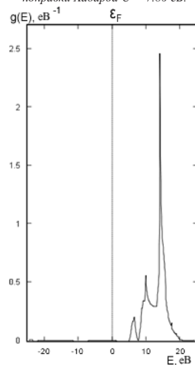
Рис. 10 – Вклад p -орбіталей атома \text{Mg} в щільність станів \text{MgO} в моделі \text{GGA} - \text{PBE} з обліком поправки Хабарда U = 7.86 \text{ eV} .
