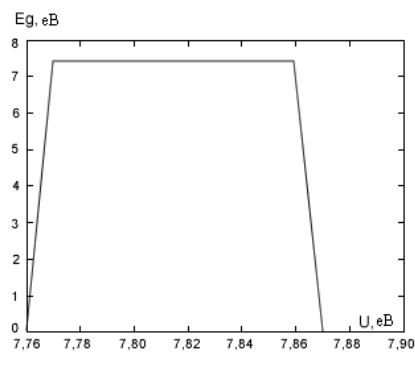
Рис. 3 – Уточнення залежності ширини E_g забороненої зони MgO в моделі GGA – PBE від параметра Хаббарда U у інтервалі 7.76 – 7.87 eV.
