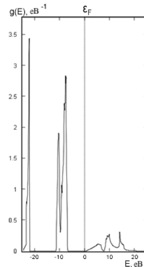
Рис. 8 – Вклад орбіталей атома \text{O} в щільність станів \text{MgO} у моделі \text{GGA} - \text{PBE} з урахуванням поправки Хабарда U = 7.86 \text{ eV} .
