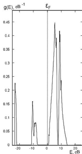
Рис. 9 – Вклад s -орбіталей атома \text{Mg} в щільність станів \text{MgO} в моделі \text{GGA} - \text{PBE} з обліком поправки Хабарда U = 7.86 \text{ eV} .
