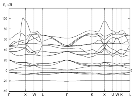
Рис. 1 – Зонна структура MgO в моделі GGA – PBE.
