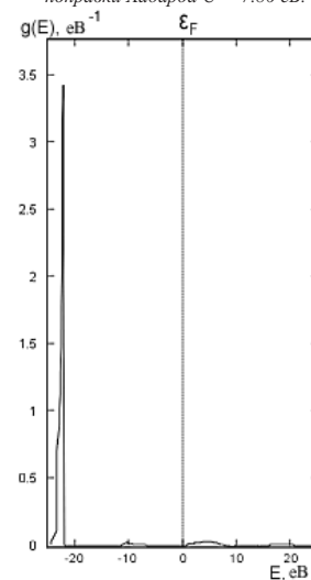
Рис. 11 – Вклад s -орбіталей атома \text{O} в щільність станів \text{MgO} в моделі \text{GGA} - \text{PBE} з урахуванням поправки Хабарда U = 7.86 \text{ eV} .
