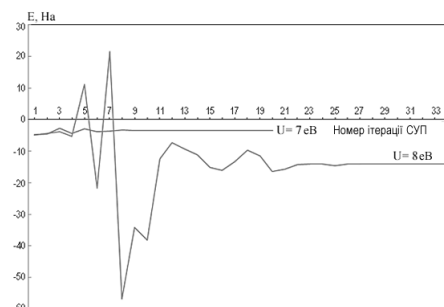
Рис. 4 – Хід процесу самоузгодження при значеннях параметра Хабарда U , рівних 7 і 8 eV, що призводить до різних електронних станів.
