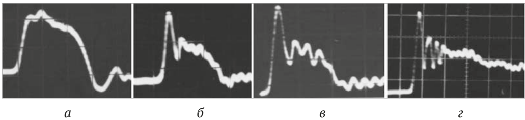
Рис. 3. Типові осцилограми взаємодії стрижня з конічною ( 2a=1700 ) (а, б, в) та плоскою головною частиною з пластиною товщиною 6 мм при швидкості удару 112 м/с (а), 141 м/с (б), 170 м/с (в), 84 м/с (г)
